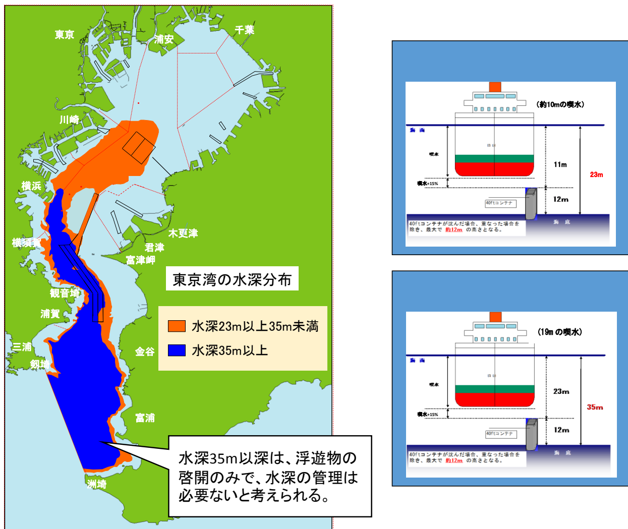
図 19 40ft コンテナが縦に沈下していた場合でも余裕水深が確保される水域
