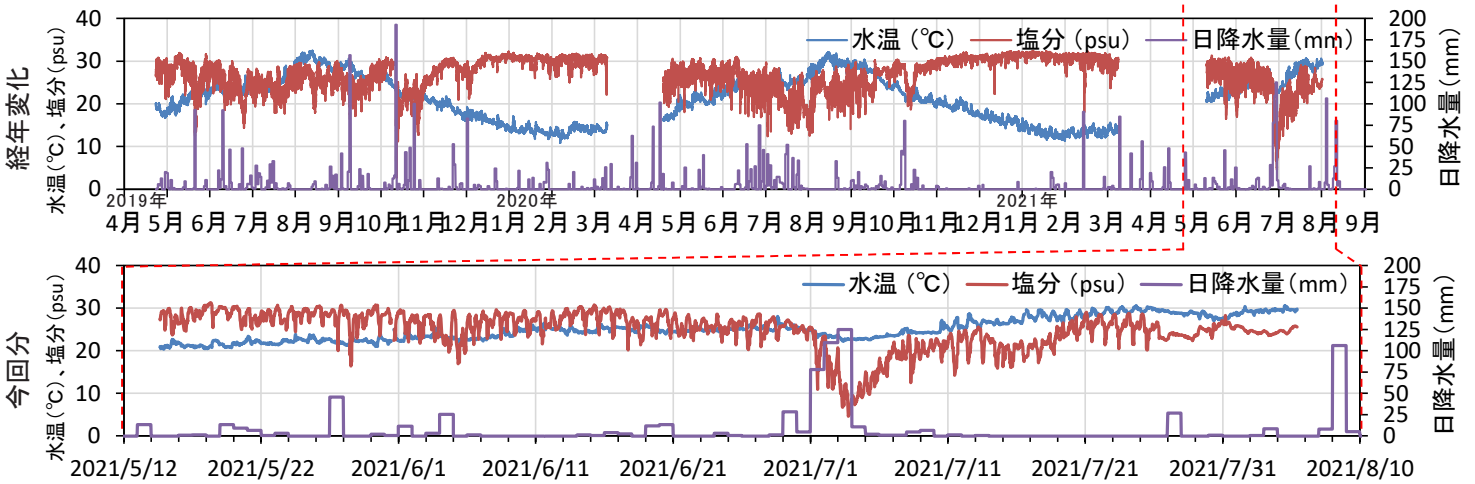
水温と塩分の測定結果と日降水量(経年変化と今回分)
