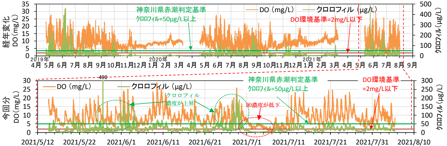
溶存酸素(DO)濃度とクロロフィル濃度の測定結果(経年変化と今回分)
